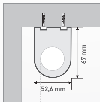
VISTA DI LATO: Attacco a soffitto.
