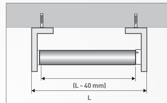
VISTA DALL'ALTO: Solo per sistema a catena. Ingombro telo: sottrarre 40 mm dalla larghezza.
