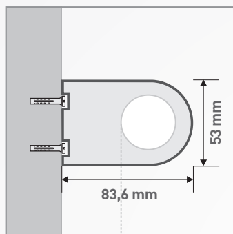
VISTA DI LATO: Attacco a parete.
