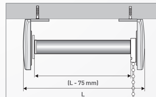
VISTA DALL'ALTO: Ingombro telo: sottrarre 75 mm dalla larghezza.
