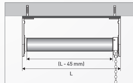
VISTA DALL'ALTO: Ingombro telo: sottrarre 45 mm dalla larghezza.
